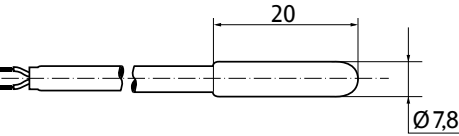
Fernfühler F 193 720 (als Zubehör)
